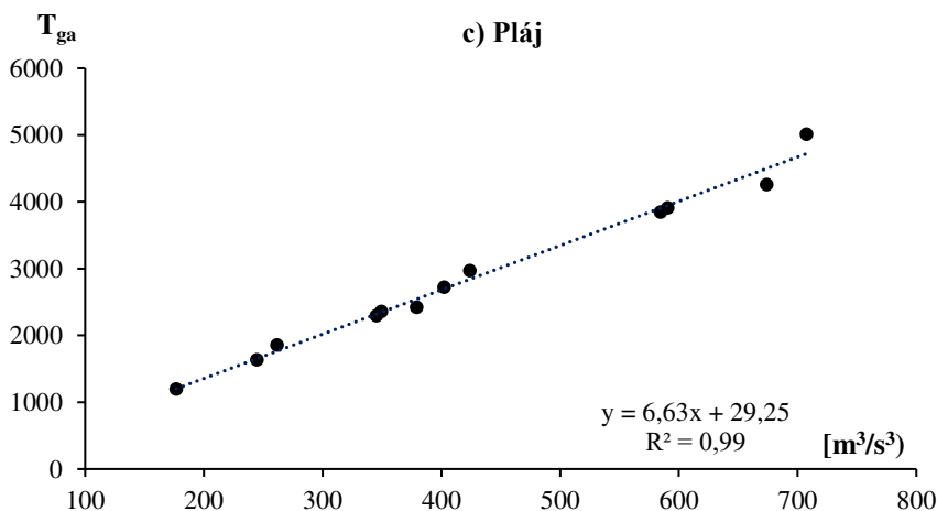
3.34. ábra. A havi átlagos fajlagos szélteljesítménnyel arányos görbe alatti terület ( T_{ga} ) és a szélesebség köbök havi átlaga ( v_m ) közötti lineáris korreláció és regresszió a) Ungvár, b) Rahó és c) Pláj állomás esetében (10 m magasságban)
