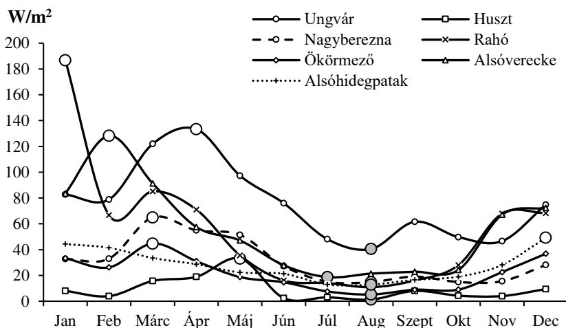
3.24. ábra. A havi átlagos fajlagos széltejesítmény (W/m 2 ) az alföldi és a folyóvölgyi állomásokon 100 m-es magasságban, 2011–2015 között (fehér kör jelölő – maximum, szürke kör jelölő – minimum érték)
