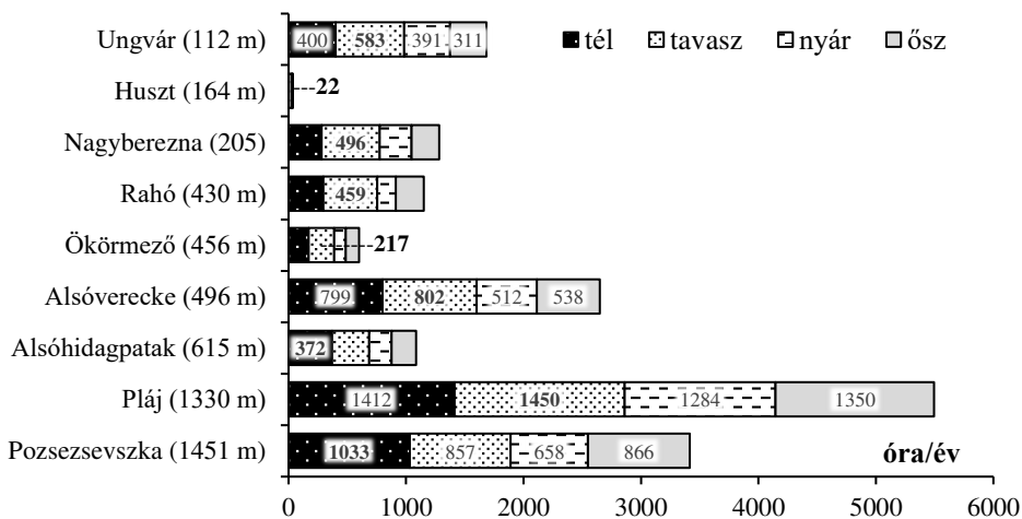
3.20. ábra. Az energetikailag hasznosítható szélsébségek időtartama (óra/évszak) 10 m-en évszakonként a 2011–2015-ös időszakban (kiemelve: a legnagyobb évszakai érték)
