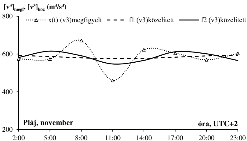
3.29. ábra. A periodikus függvény „legrosszabb” illeszkedése a szélsébséghöbök napi menetére
