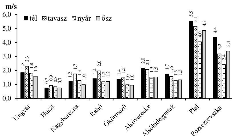
3.1. ábra. Az évszakos átlagos szélsőbesség (m/s) alakulása 2011–2015 között Forrás: saját szerkesztés
