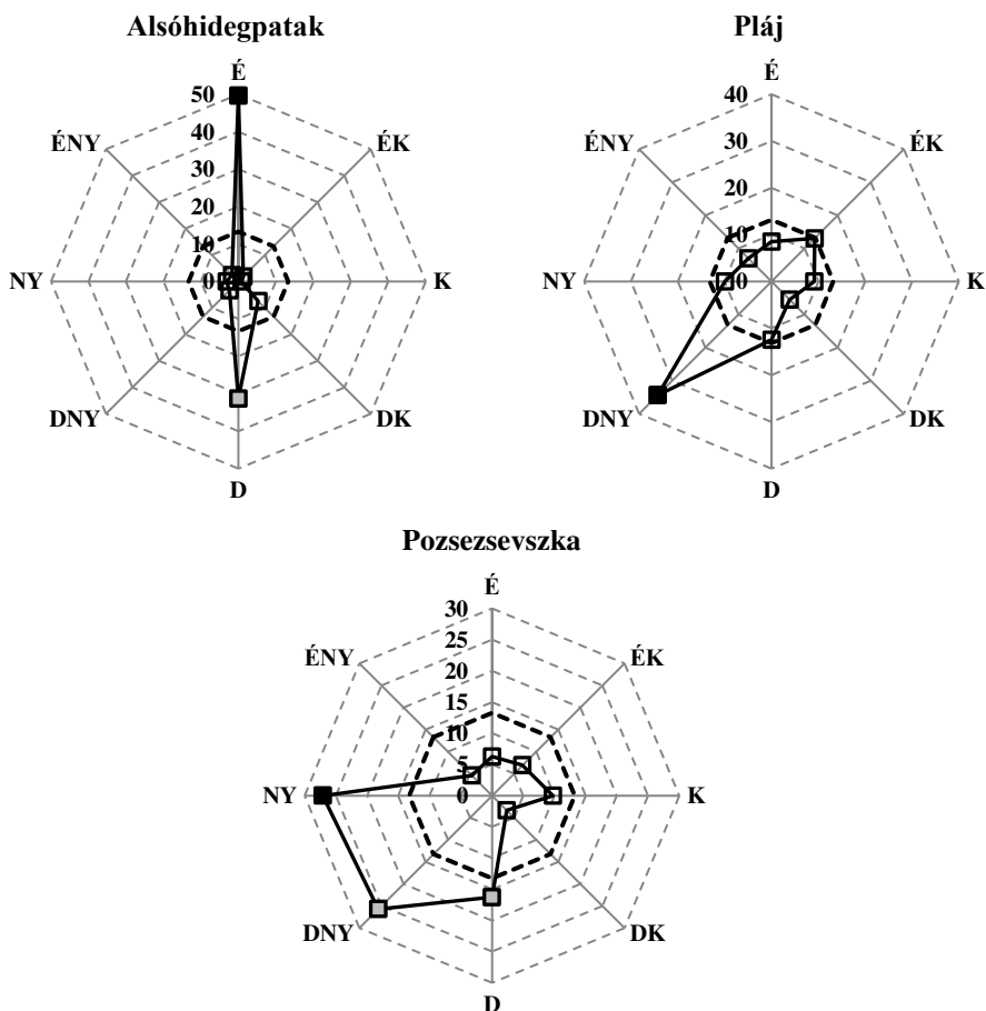
3.36. ábra. A szélirányok relatív gyakorisága (%) és a jellemző szélirányok a vizsgált állomásokon a 2011–2015 közötti időszakban (feketével kitöltött jelölő – a leggyakoribb jellemző szélirány, szürkével kitöltött jelölők – a többi jellemző szélirány, fekete szaggatott vonal – kritikus gyakorisági érték ( h_2 ), amely fölött az adott szélirány jellemzőnek tekinthető, szürke vonal – szélrózsza)
