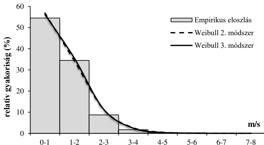
3.12. ábra. Ökörmező napi átlagos szélesebbeségeinek relatív gyakorisági eloszlása és az arra szignifikáns illeszkedést adó elméleti eloszlások 2011–2015 között
