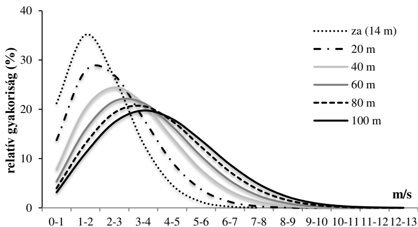
3.15. ábra. A napi átlagos szélesebségek relatív gyakorisági eloszlása Ungváron az anemométer magasságában ( z_a ) és további 5 szinten (2011–2015)
