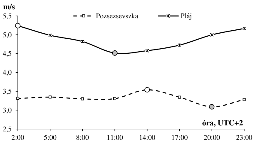
3.8. ábra. A hegyes Pozsezevszka és a Pláj állomások terminus időpontokénti átlagos szélsőségeinek (m/s) napi menete 2011–2015 között (fehér kör jelölő – maximum, szürke kör jelölő – minimum érték)
