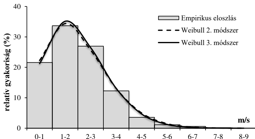
3.11. ábra. Ungvár napi átlagos szélesebbeségeinek relatív gyakorisági eloszlása és az arra szignifikáns illeszkedést adó elméleti eloszlások 2011–2015 között
