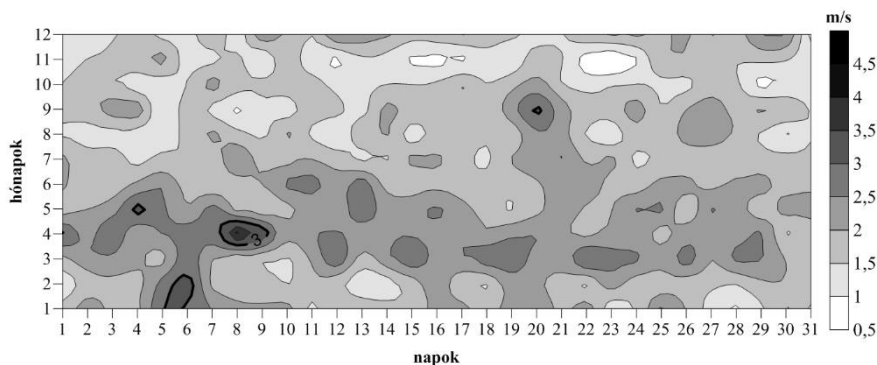
3.3. ábra. Ungvár napi átlagos szélesebségének (m/s) éves menete 2011–2015 között
