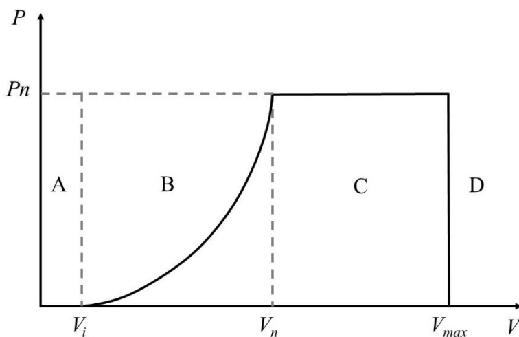
3.19. ábra. A szél erőművek jellemző szélesebbesség-teljesítmény görbéje
