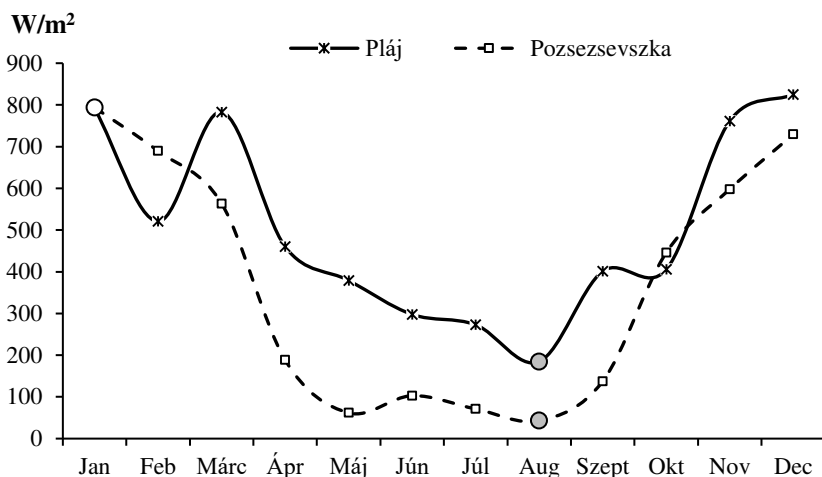
3.26. ábra. A havi átlagos fajlagos szélteljesítmény ( \text{W/m}^2 ) a hegységi állomásokon 100 m-es magasságban, 2011–2015 között (fehér kör jelölő – maximum, szürke kör jelölő – minimum érték)
