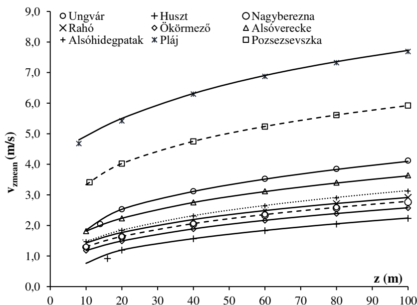
3.18. ábra. Az egész mérési időszakra számított átlagos szélesebességek (pontok) és a rájuk illesztett hatványfüggvény (vonalak)
