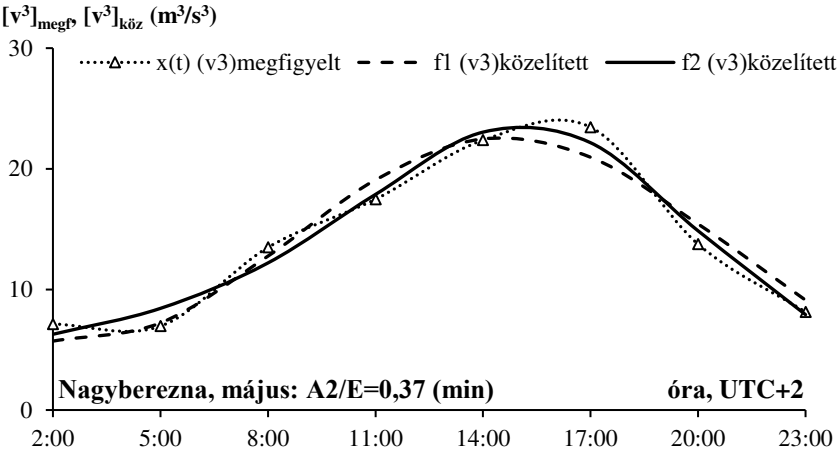
3.32. ábra. A szélesebbesség köbök óraátlagainak közelítése napi egy- és kétperiódusú hullámmal igen gyenge 2. hullám (félnapos periódusú) esetén Forrás: saját szerkesztés
