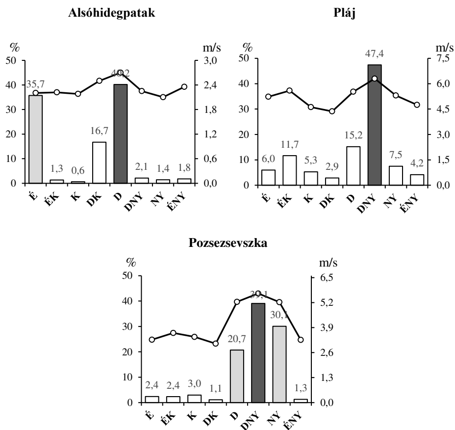
3.38. ábra. A különböző szélirányok relatív energiatartalma (%), azok átlagsebessége (m/s, fekete vonal jelölőkkel), az energetikailag uralkodó szélirány (fekete oszlop) és a többi jellemző szélirány (szürke oszlopok), 2011–2015 között
