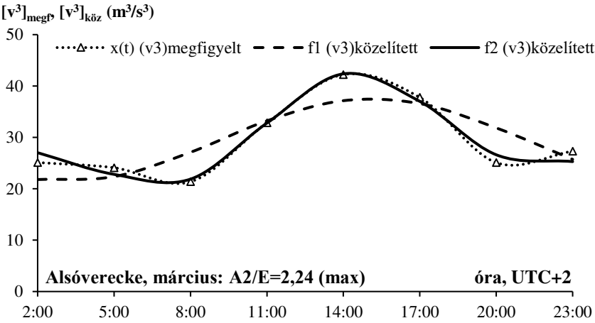
3.33. ábra. A szélesebbesség köbök óraátlagainak közelítése napi egy- és kétperiódusú hullámmal igen erős 2. hullám (félnapos periódusú) esetén Forrás: saját szerkesztés
