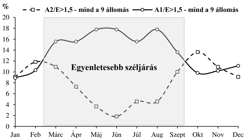
3.31. ábra. Az egynapos ( A_1/E > 1,5 ) és a félnapos periódusú hullám ( A_2/E > 1,5 ) realitásának havi gyakoriságai (%-ban), p=0,17 szignifikancia szinten mind a 9 állomáson
