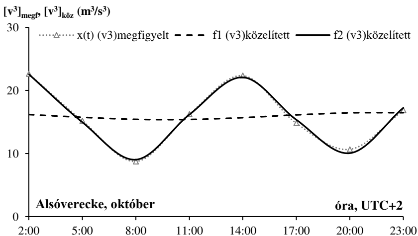
3.28. ábra. A periodikus függvény „legjobb” illeszkedése a szélsébséghöbök napi menetére
