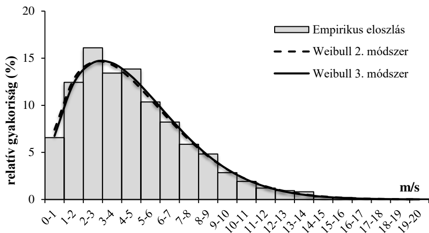
3.13. ábra. Pláj napi átlagos szélesebbeségeinek relatív gyakorisági eloszlása és az arra szignifikáns illeszkedést adó elméleti eloszlások 2011–2015 között
