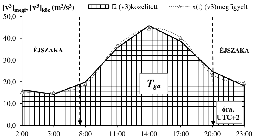
3.27. ábra. A szélsébség köb (m³/s³) átlagok számolt és a közelítő függvénynel előállított értékeinek napi menete Forrás: saját szerkesztés
