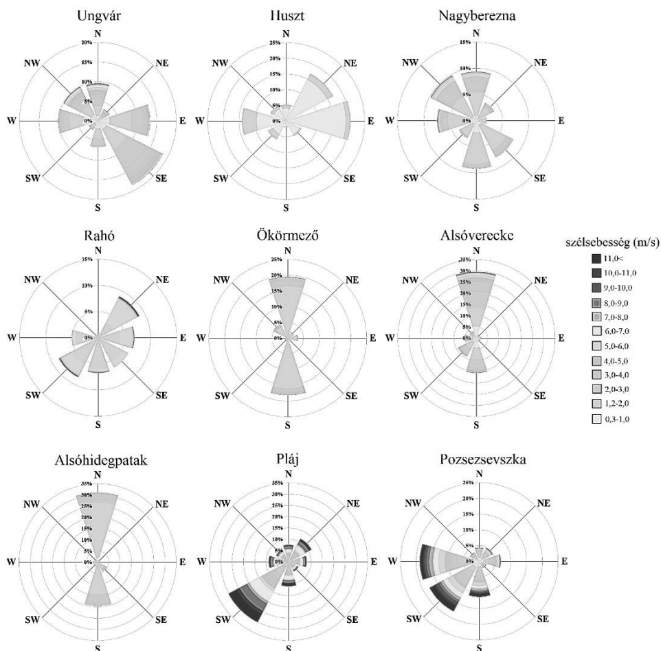
3.37. ábra. A szélirányszektorokhoz tartozó szélesség eloszlás (%) az egyes állomásokon a 2011–2015 közötti időszakban
