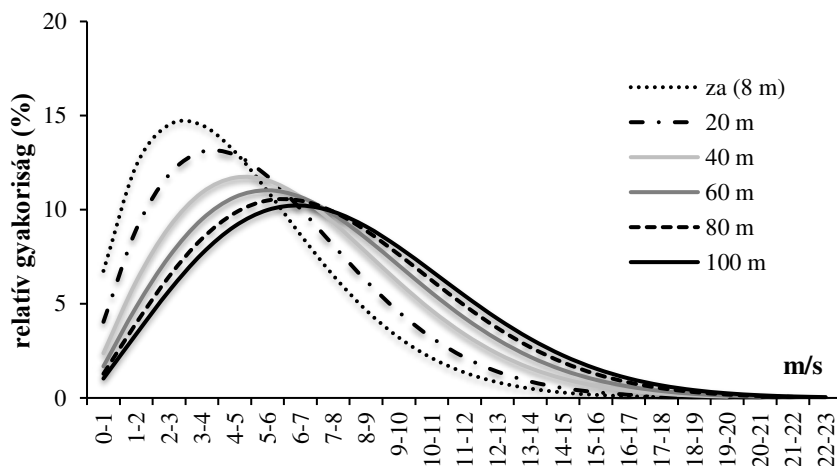
3.17. ábra. A napi átlagos szélesebségek relatív gyakorisági eloszlása a Plájon az anemométer magasságában ( z_a ) és további 5 szinten (2011–2015)
