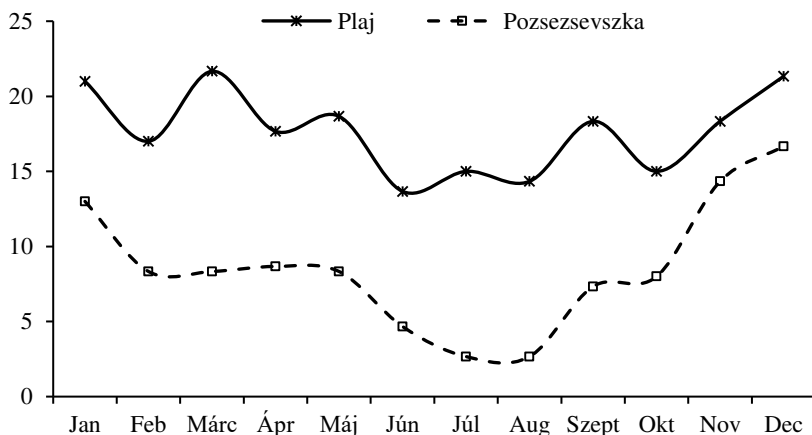
3.10. ábra. A szeles napok (D10) havonkénti átlagos száma 2013–2015 között a hegységi Pláj és a Pozsezevszka állomásokon
