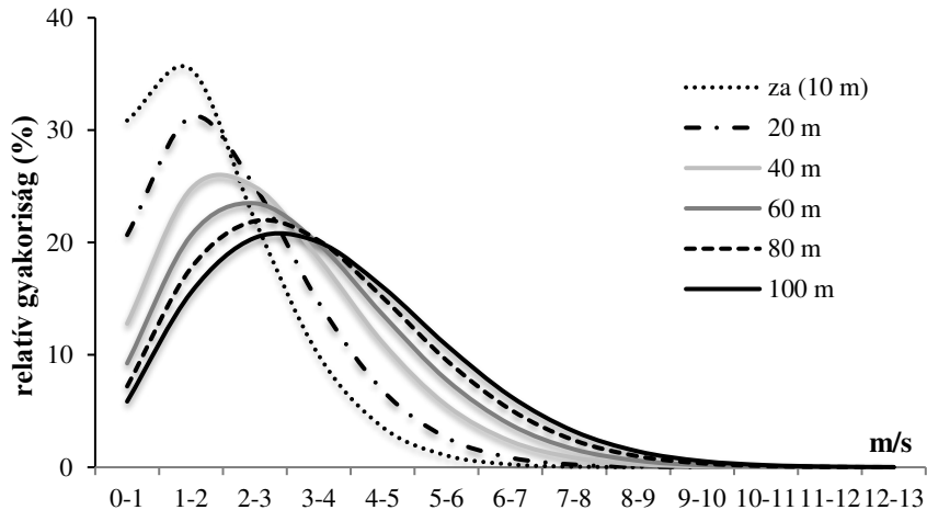
3.16. ábra. A napi átlagos szélesebségek relatív gyakorisági eloszlása Alsóvereckén az anemométer magasságában ( z_a ) és további 5 szinten (2011–2015)
