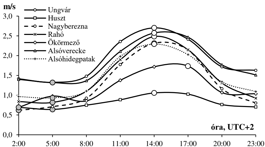
3.7. ábra. Az alföldi és nem alföldi folyóvízgyi állomások terminus időpontokénti átlagos szélsőségeinek (m/s) napi menete 2011–2015 között (fehér kör jelölő – maximum, szürke kör jelölő – minimum érték)
